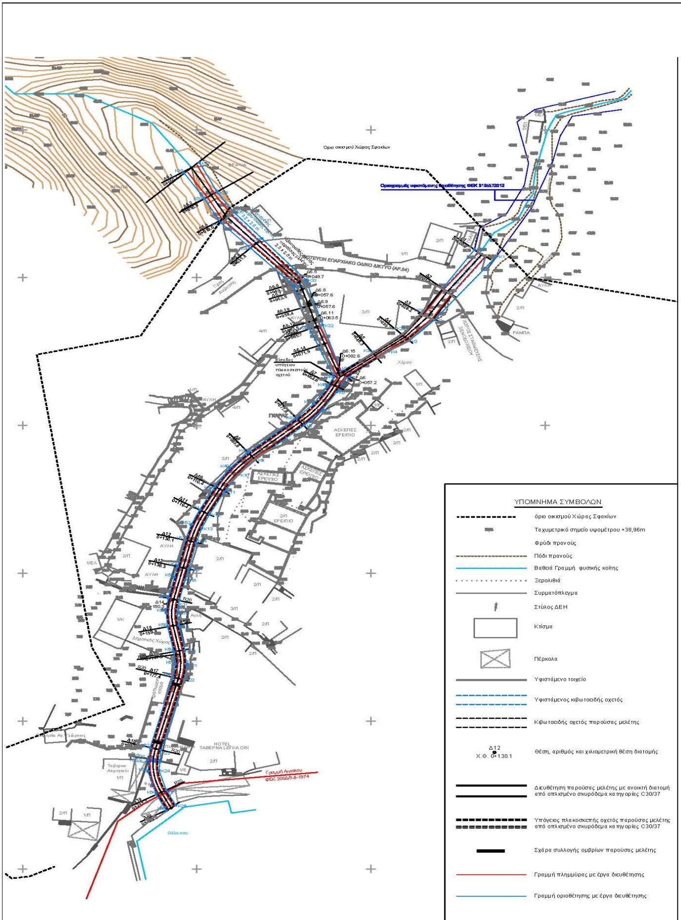
Εικόνα 1 Γενική διάταξη έργων οριοθέτησης_Απόσπασμα σχεδίου 12
