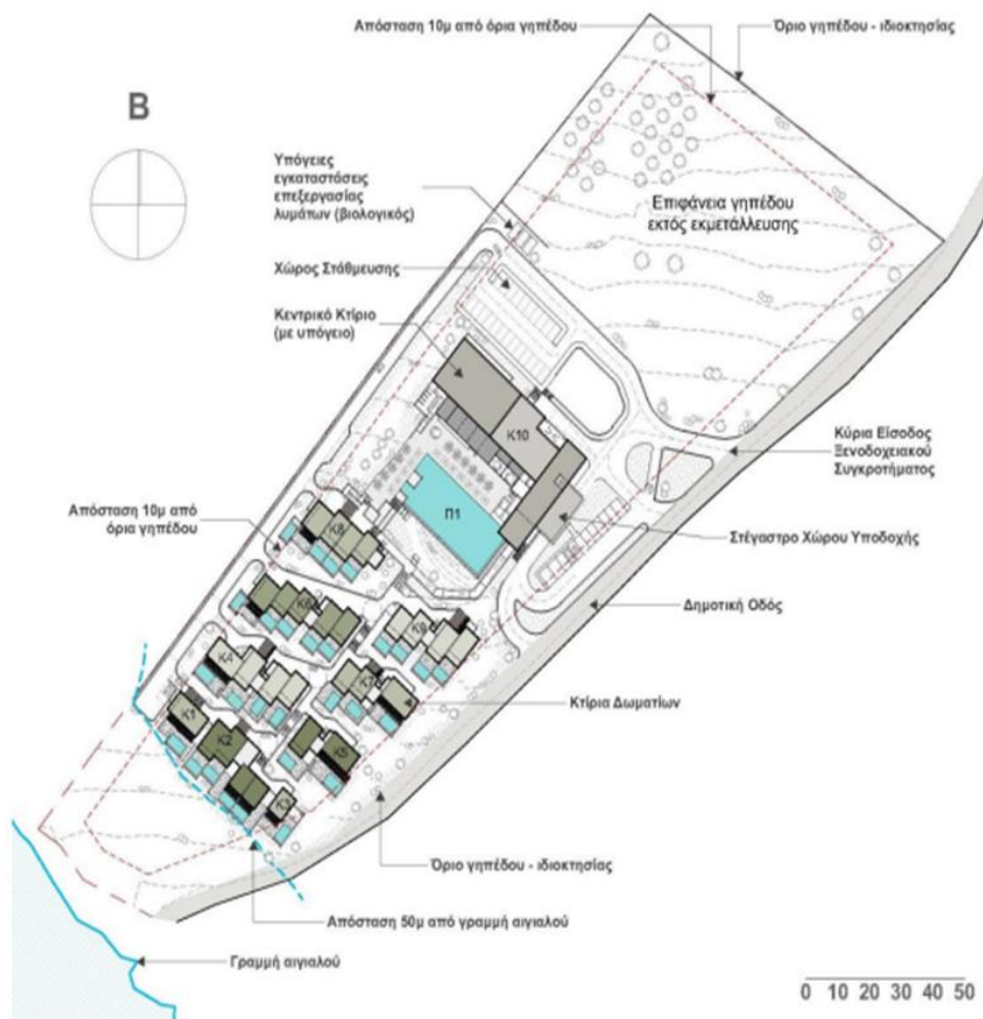
Εικόνα 6-1 Γενική διάταξη έργου
