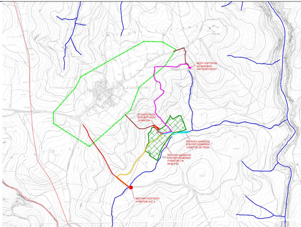
Εικόνα 1. Θέση ΕΕΛ, αντλιοστασίων, αγωγών ακαθάρτων, επεξεργασμένων και τελική διάθεση.
