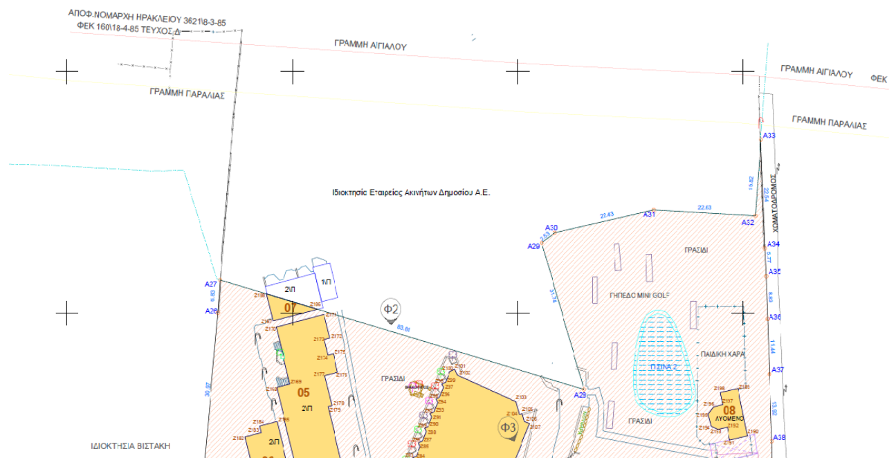
Εικόνα 2: Τμήμα Τοπογραφικού Διαγράμματος
