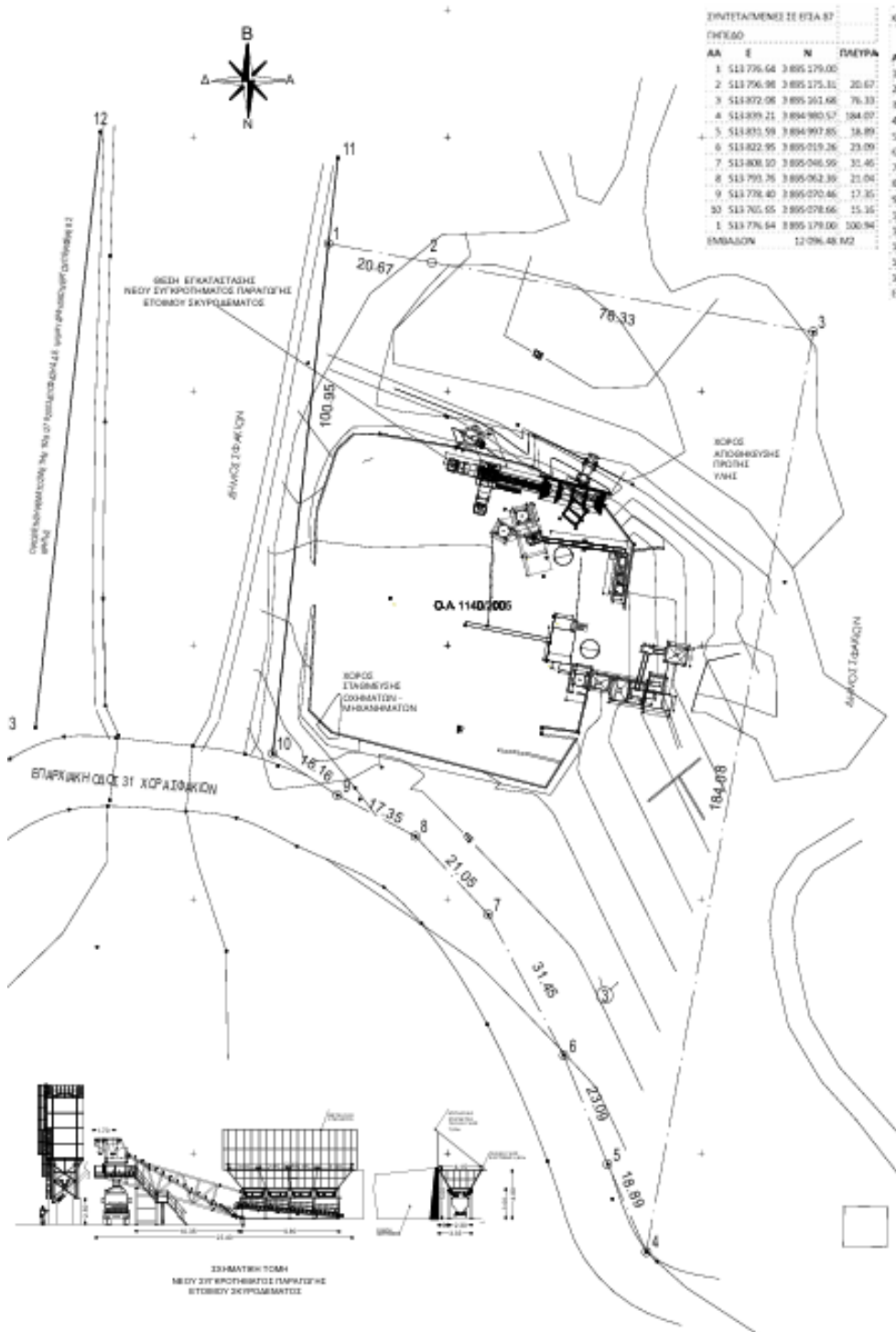
Εικόνα 6. Απόσπασμα από το Διάγραμμα κάλυψης (ΜΠΕ-2) της δραστηριότητας «ΣΥΓΚΡΟΤΗΜΑ ΠΑΡΑΓΩΓΗΣ ΑΔΡΑΝΩΝ ΥΛΙΚΩΝ ΚΑΙ ΕΤΟΙΜΟΥ ΣΚΥΡΟΔΕΜΑΤΟΣ (ΥΦΙΣΤΑΜΕΝΟΥ ΚΑΙ ΝΕΟΥ) ΙΩΑΝΝΗΣ ΧΑΤΖΗΔΑΚΗΣ ΚΑΙ ΣΙΑ Ο.Ε.» στη θέση «Ξηροτόταμος» Δήμου Σφακίων Χανίων.
