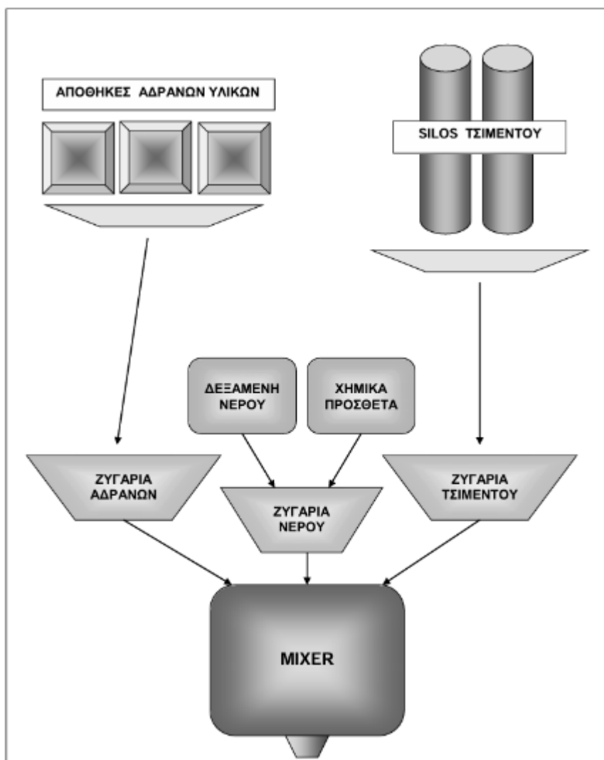
Εικόνα 5. Διάγραμμα παραγωγής έτοιμου σκυροδέματος (σελ. 87 της ΜΠΕ) της δραστηριότητας του έργου «ΣΥΓΚΡΟΤΗΜΑ ΠΑΡΑΓΩΓΗΣ ΑΔΡΑΝΩΝ ΥΛΙΚΩΝ ΚΑΙ ΕΤΟΙΜΟΥ ΣΚΥΡΟΔΕΜΑΤΟΣ (ΥΦΙΣΤΑΜΕΝΟΥ ΚΑΙ ΝΕΟΥ) ΙΩΑΝΝΗΣ ΧΑΤΖΗΔΑΚΗΣ ΚΑΙ ΣΙΑ Ο.Ε.» στη θέση «Ξηροπόταμος» Δήμου Σφακίων Χανίων.
